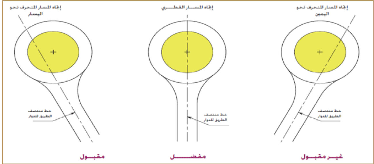
شكل 27: التخطيط القطري لمسارات الطرق المقترية من مدخل الدوار
