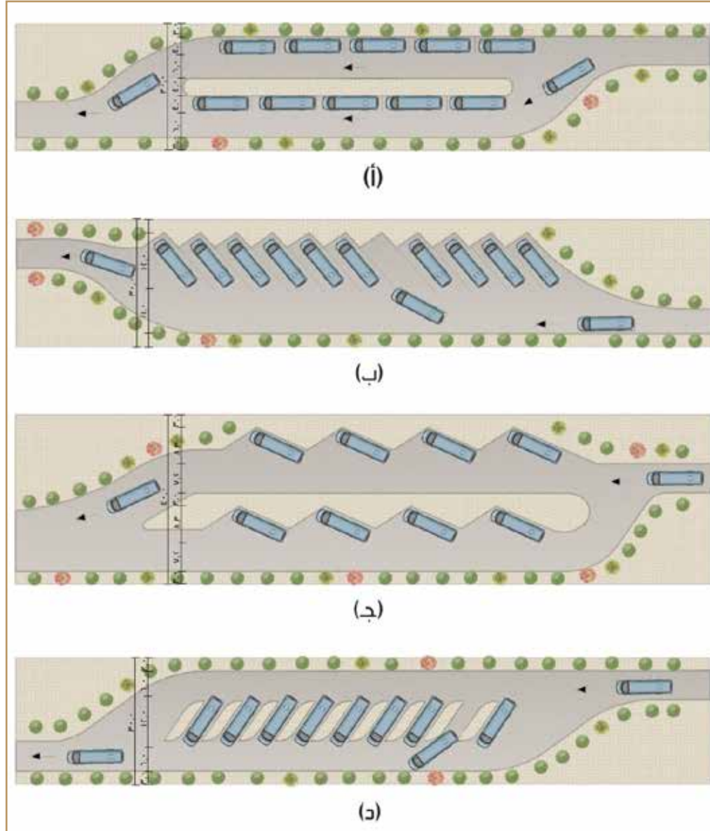
شكل 35: أنماط مختلفة من ساحات وقوف الحافلات (بالمتر)
