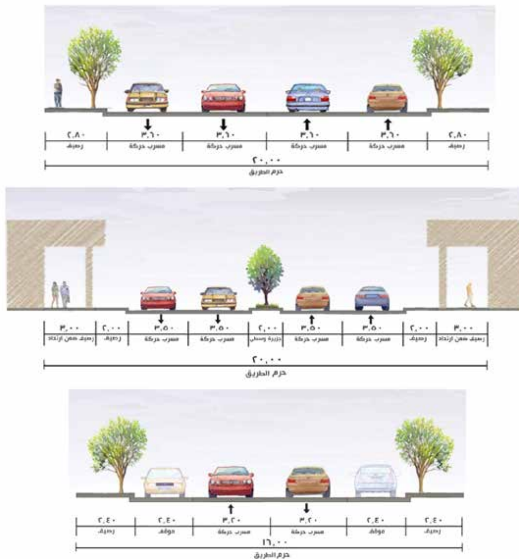
شكل 3 (تتمة): مقاطع عرضية متعددة لطرق شريانية في المنطقة الحضرية لأبعاد مختلفة من حرم الطريق
