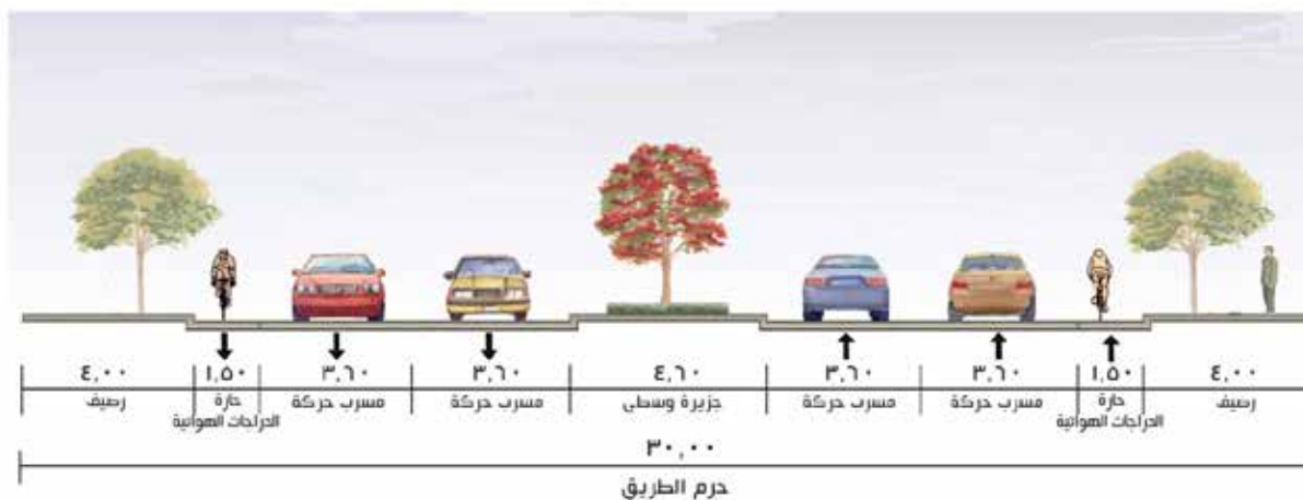
شكل 6: مقطعين عرضيين نموذجيين يشملان حارة أو حارتين للدراجات الهوائية
