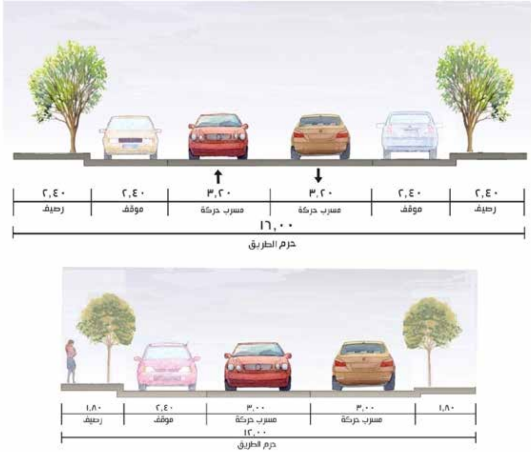
شكل 4: مقاطع عرضية متعددة لطرق تجميعية في المنطقة الحضرية لأبعاد مختلفة من حرم الطريق
