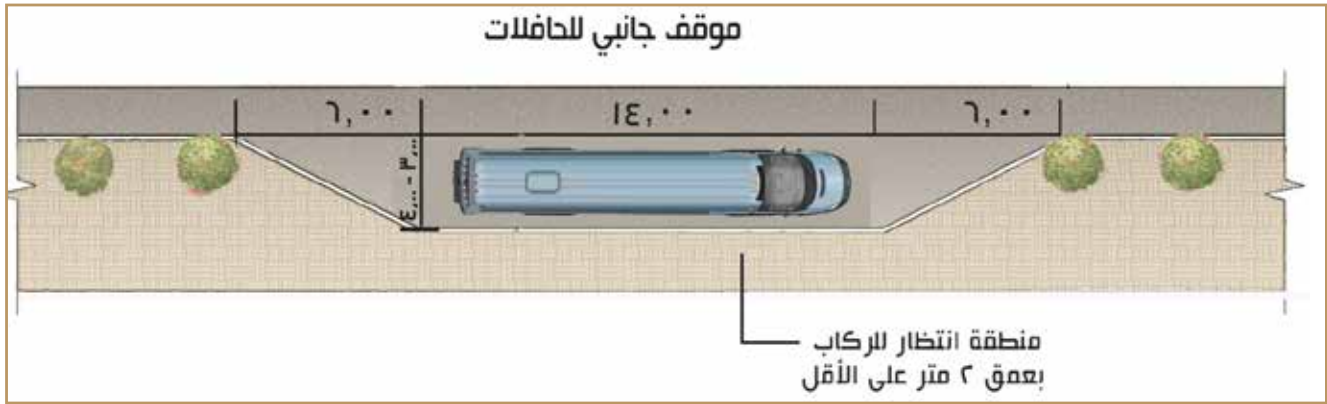
شكل 34: نموذج لموقف جانبي للحافلات مواز لمسار الحركة (بالمتر)
