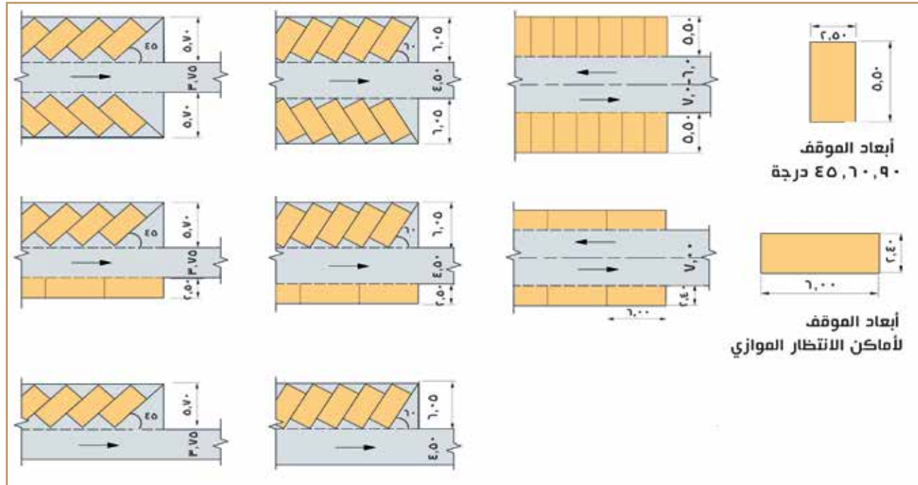
شكل 33: أنماط مختلفة من تخطيط ساحات وقوف السيارات (بالمتر)
