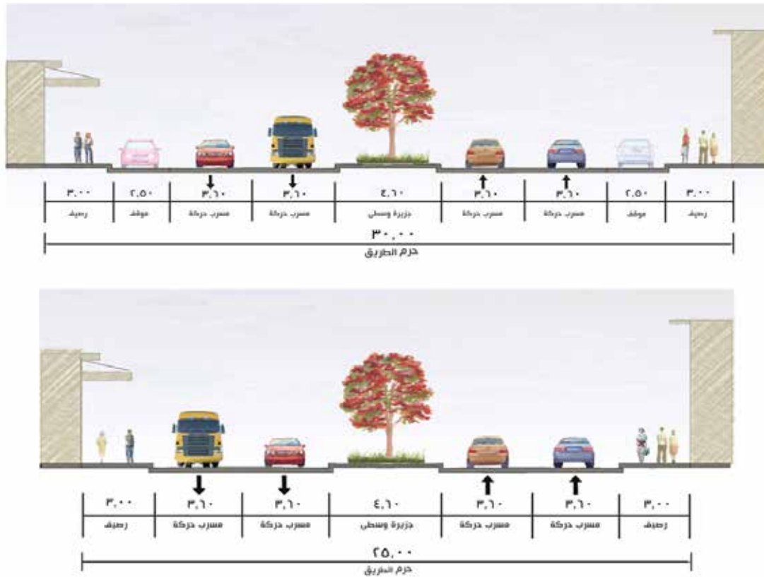
شكل 3: مقاطع عرضية متعددة لطرق شريانية في المنطقة الحضرية لأبعاد مختلفة من حرم الطريق
