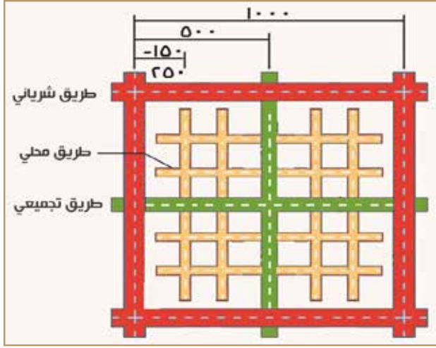
شكل 45: نموذج يبين التباعد بين التقاطعات (بالمتر)
