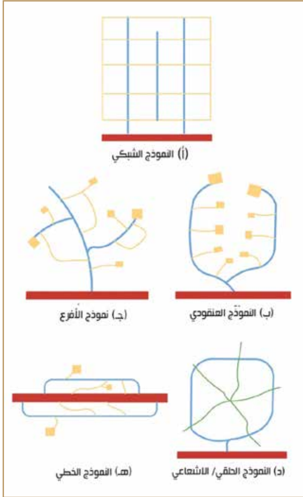
شكل 38: رسوم توضيحية لنماذج تخطيط شبكات الطرق
