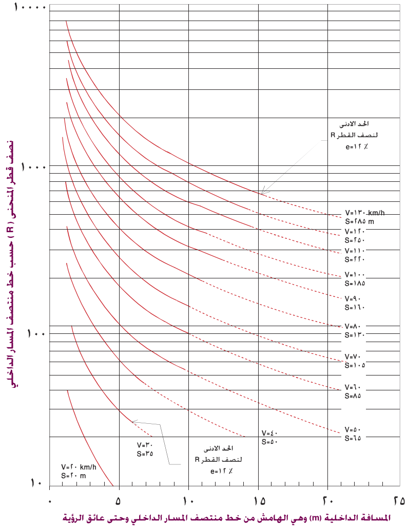
شكل 14: مسافة الهامش (m) حسب نصف قطر المنحني (R) وسرعة التصميم (أو مسافة الرؤية اللازمة للتوقف)
