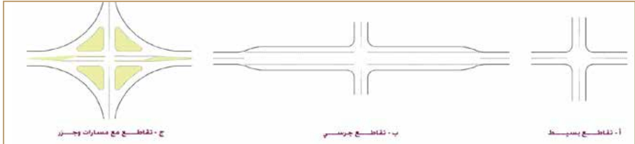
شكل 17: نماذج لأنواع مختلفة من التقاطعات ذات الأذرع الأربعة للطرق المتقاطعة على زاوية قائمة
