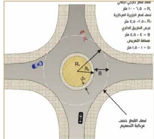
شكل 28: تصميم الدوار الصغير
