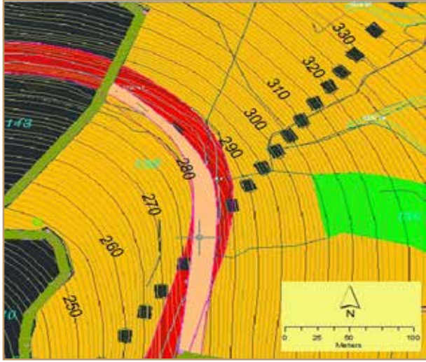
شكل 41: اختيار موقع الطريق مع الأخذ بالاعتبار طبوغرافيا المنطقة
