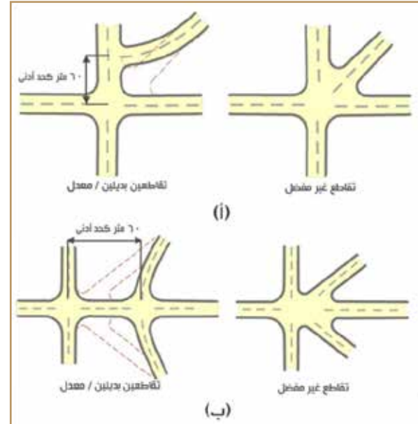
شكل 18: إعادة توجيه طريق أو أكثر عند تقاطع متعدد الأذرع
