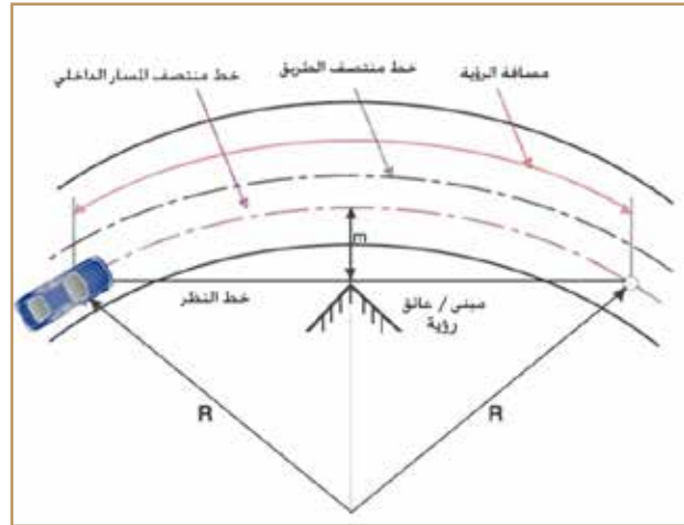
شكل 13: مسافة الرؤية اللازمة للتوقف على منحنى أفقي
