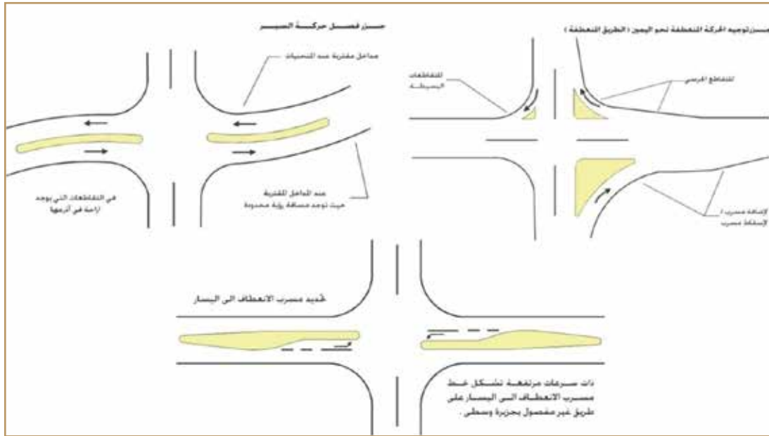
شكل 23: أمثلة على عملية توجيه الحركة على التقاطعات والجزر
