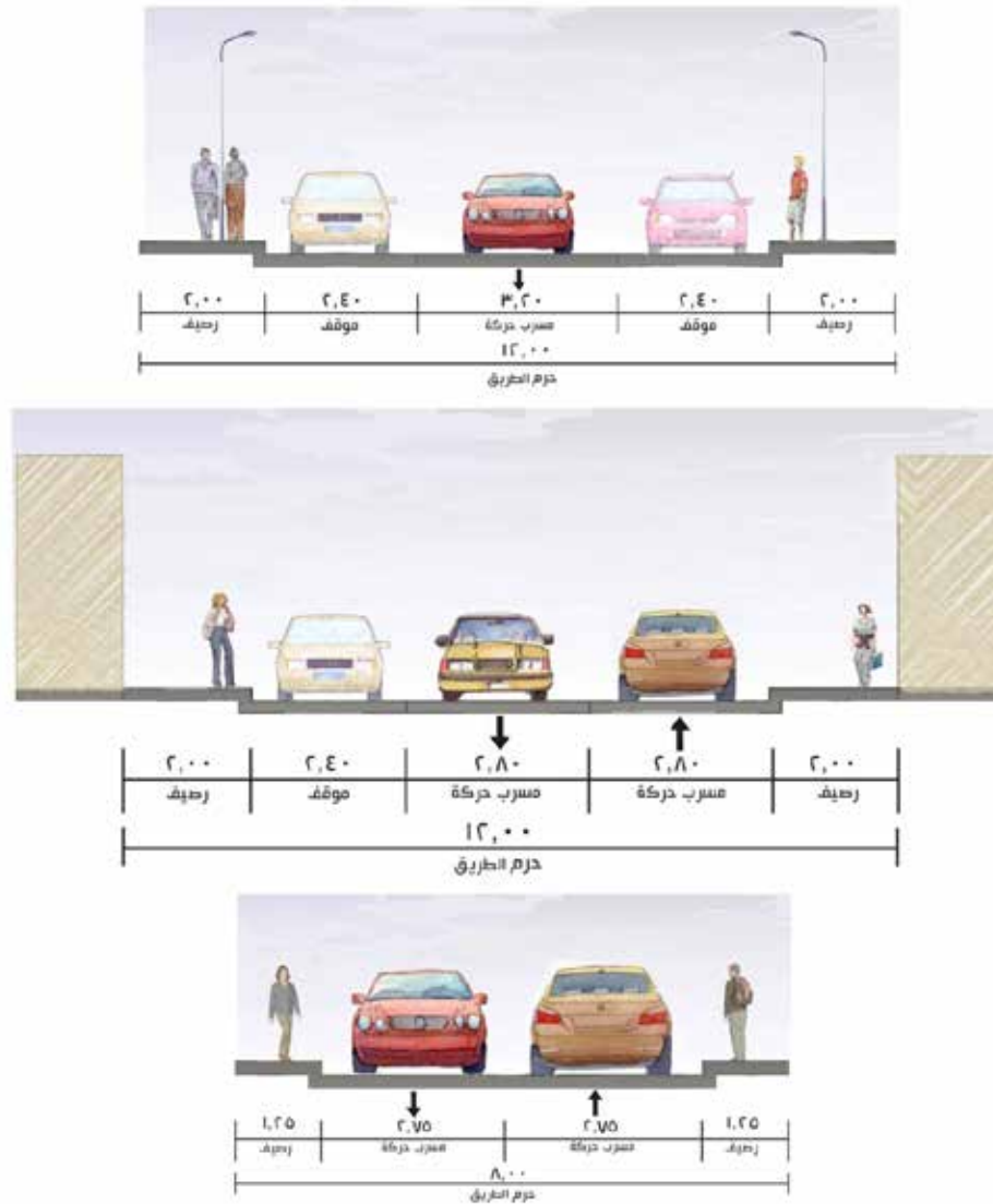
شكل 5: مقاطع عرضية متعددة لطرق محلية في المنطقة الحضرية لأبعاد مختلفة من حرم الطريق
