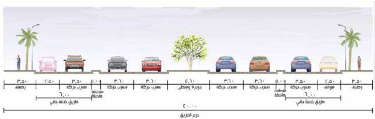
شكل 10: مقطع عرضي نمذجي على طريق خدمة جانبي على كل من جانبي الطريق
