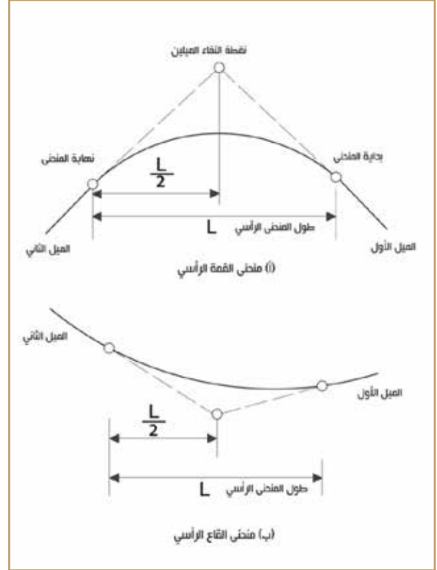
شكل 15: رسمان توضيحيان يبينان منحنيات القمة أو القاع الرأسية
